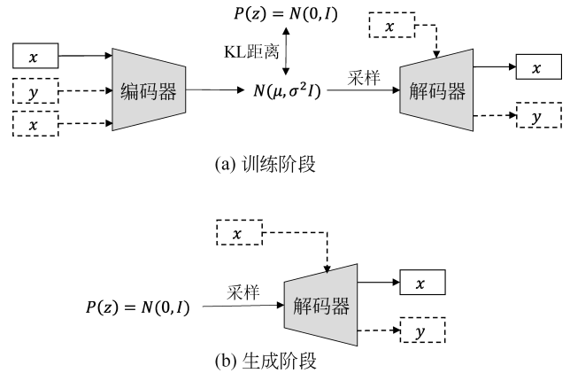
图2 变分自编码器训练和生成过程
