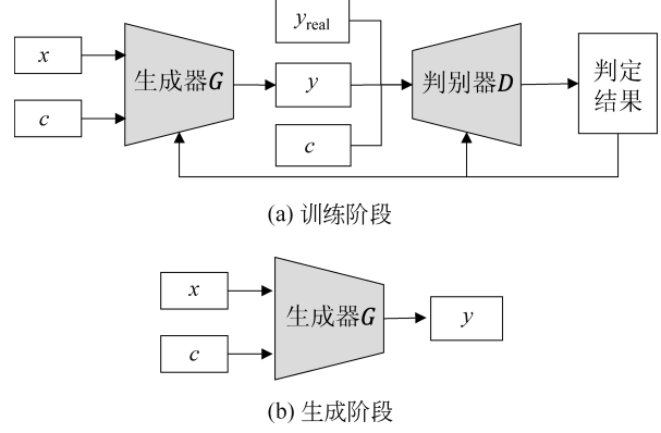
图 1 生成对抗网络在可控文本生成时的训练和生成过程
